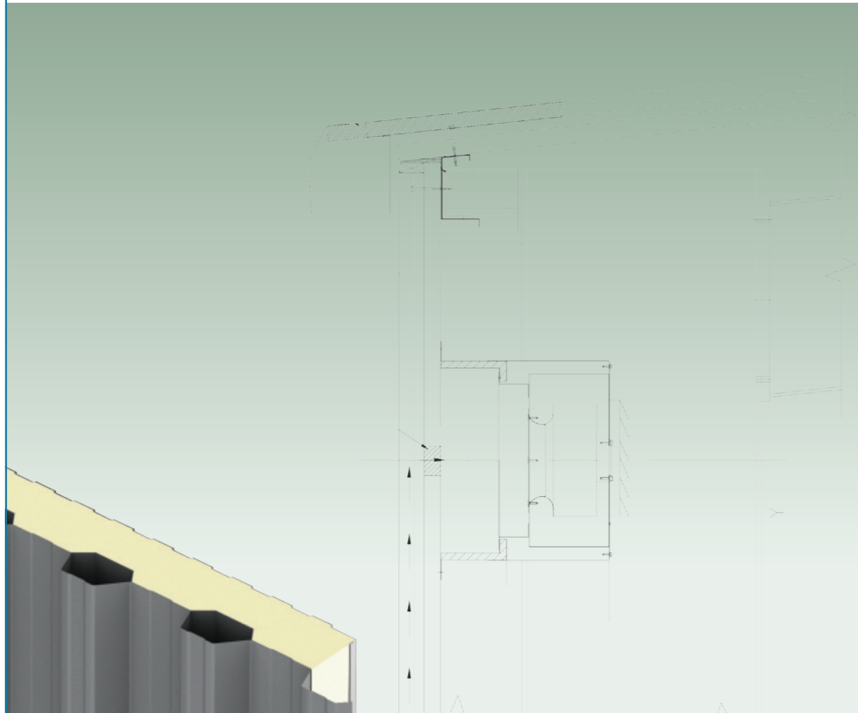
Principe werking EnergiPanel; De temperatuur van de getransporteerde lucht loopt op tot 80 °C
